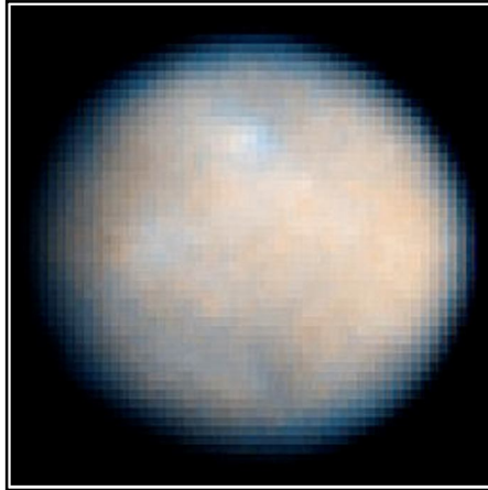
(Aufnahme: hubble-Teleskop)
