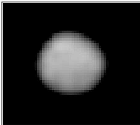
(Aufnahme: hubble-Teleskop)
